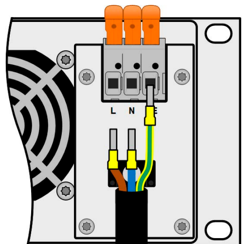
Bild 9 - Beispielkonfiguration eines AC-Kabels
