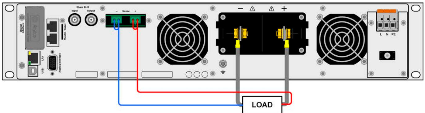
Bild 12 - Beispiel Fernfühlungsverdrahtung (DC- und Sense-Abdeckungen zu Zwecken der Veranschaulichung weggelassen)
