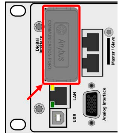
Bild 3 - Schnittstellenlot
