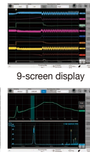
FFT display
