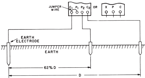
Abb. 11: Spannungsabfall- oder Dreileiterverfahren für
