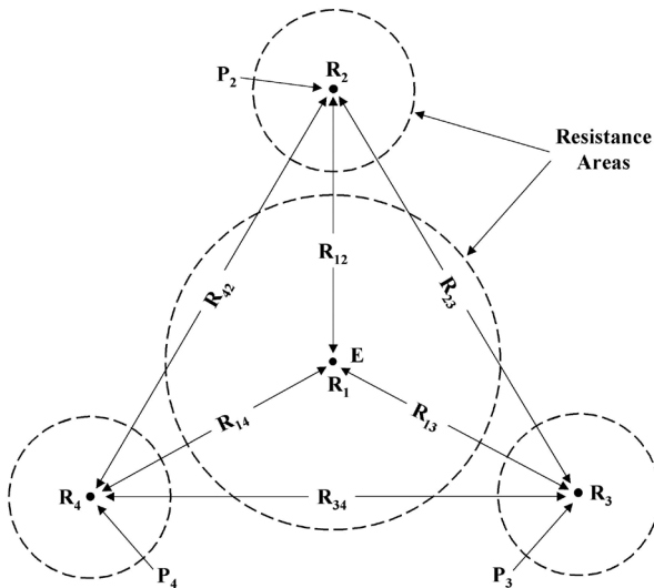
Abb. 33: Stern-Dreieck-Prüfaufbau
