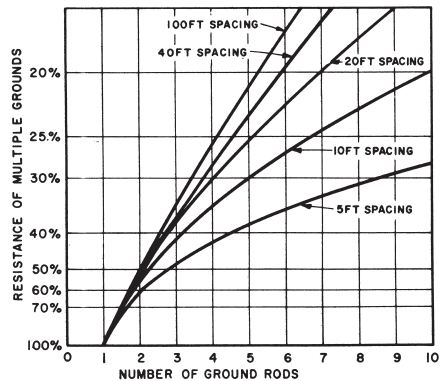
Abb. 18: Vergleichswiderstände von Erdungselektroden mit mehreren Stäben Ein Stab entspricht 100 % 9
