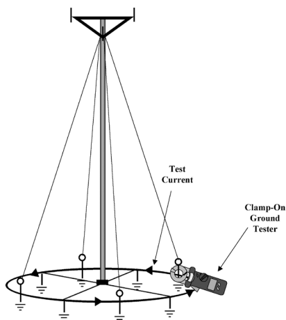
Abb. 24: Mobilfunkmast – Beispiel einer falsch eingesetzten Anwendung
