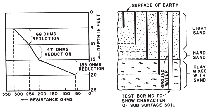
Abb. 3: Tiefere Erdelektroden verringern den Widerstand. Diese Diagramme zeigen den Zusammenhang zwischen dem Bodentyp und dem Widerstand der eingeführten Elektrode in größeren Tiefen.
