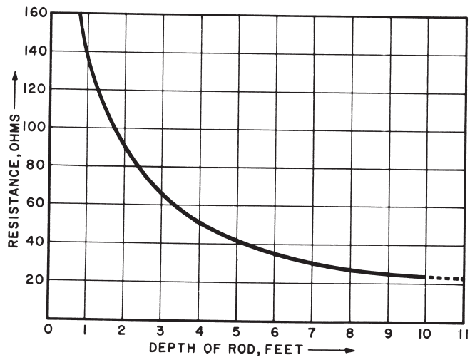
Abb. 15: Erdungswiderstand nimmt mit der Tiefe der Elektrode in der Erde ab (Quelle: Ref. 19) Sie
