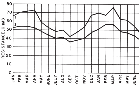
Abb. 4: Jahreszeitlich bedingte Schwankungen des Erdungswiderstandes mit einer Elektrode aus einem 3/4"-Rohr in steinigem Tonboden. Die Tiefe der Elektrode in der Erde beträgt 3 Fuß für Kurve 1 und 10 Fuß für Kurve 2 (Quelle: Referenz 9, Seite 76)
