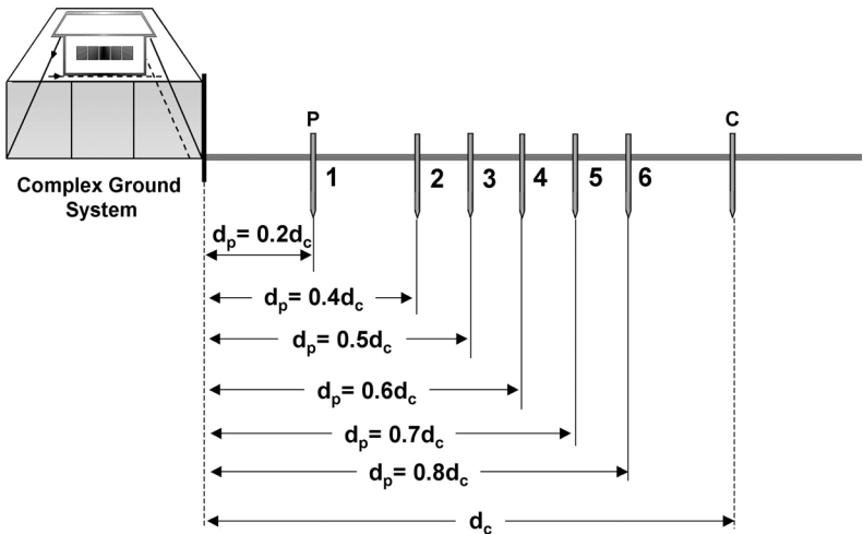
Abb. 32: Prüfaufbau für die Vierleitermethode
