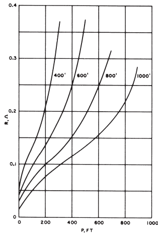
Abb. 29: Erdungswiderstandskurven für eine Umspannstation
