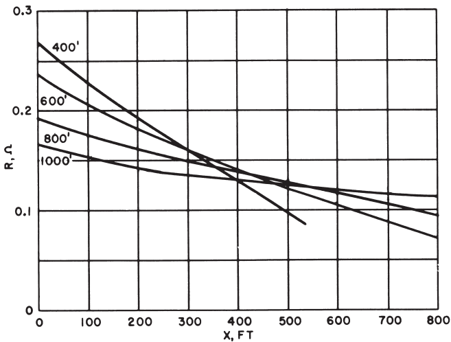
Abb. 30: Schnittkurven für Abb. 29 Die Mitte des Dreiecks, das durch die Überschneidung in Abb. 30 gebildet wird, zeigt einen Erdungswiderstand von 0,146 Ω
