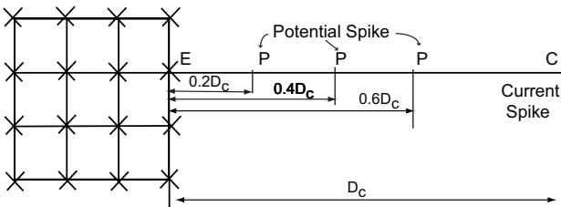
Abb. 31: Positionen für den Spannungsmessabgriff bei der Anstiegsmethode
