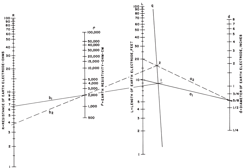
Abb. 21: Nomogramm der grundlegenden Einflussfaktoren des Erdungswiderstandes
