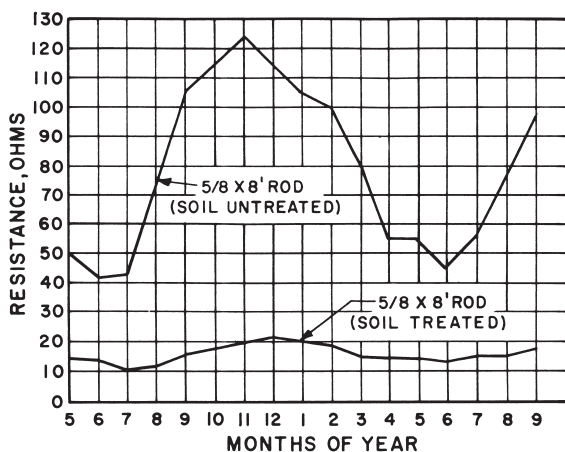
Abb. 20: Die chemische Behandlung des Bodens vermindert saisonale Schwankungen des Erdungswiderstandes der Elektroden. 11
