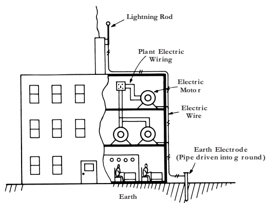
Abb. 6: Vereinfachtes Erdungssystem in einer Industrieanlage
