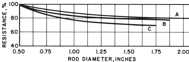
Abb. 16: Durchmesser eines Stabes hat wenig Einfluss auf seinen Erdungswiderstand
