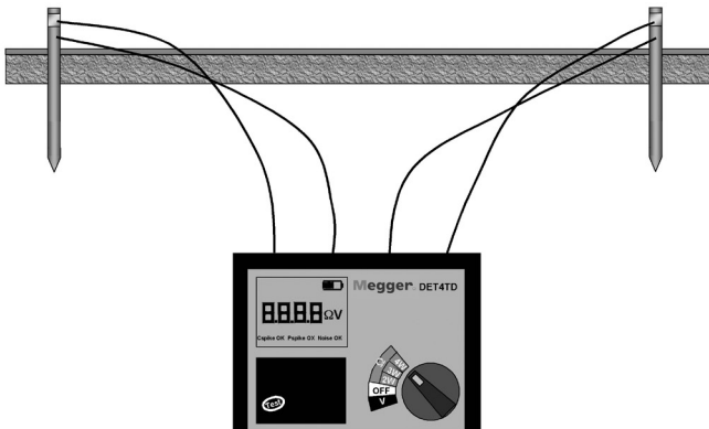
Abb. 34: Durchführung einer Zweipunktmessung
