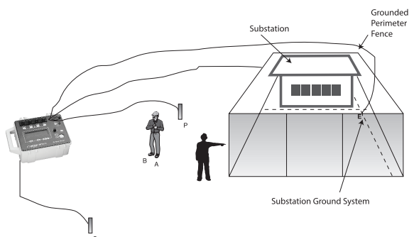
Abb. 35: Methode zur Bestimmung der Berührungs- und Schrittspannung
