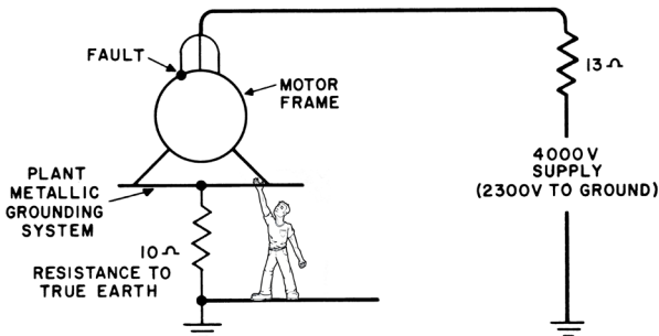
Abb. 7: Beispiel für eine elektrische Schaltung mit zu hohem Erdungswiderstand
