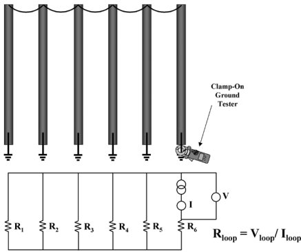
Abb. 23: Polerdungsanwendungen
