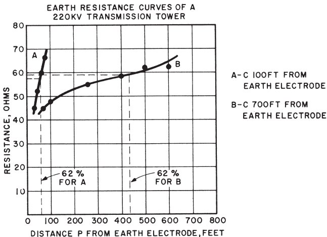
Abb. 14: Beispiel für den Einfluss der Position von C auf die Erdungswiderstandskurve
