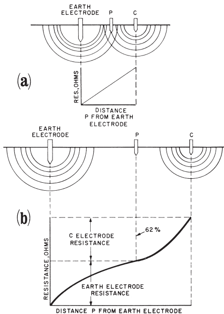
Abb. 13: Auswirkung der Position von C auf die Erdungswiderstandskurve
