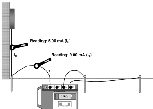
Abb. 26: Messung des Ableitstroms
