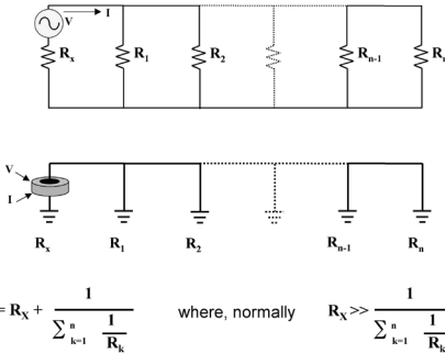
Abb. 22: Grundlegende Clamp-on-Verfahren für Erdungsprüfungen
