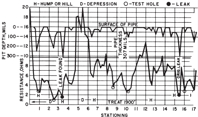
Abb. 2: Die Erdungswiderstandsprüfung der Pipeline zeigt, wo Korrosion am wahrscheinlichsten auftritt (Quelle: Referenz 18)
