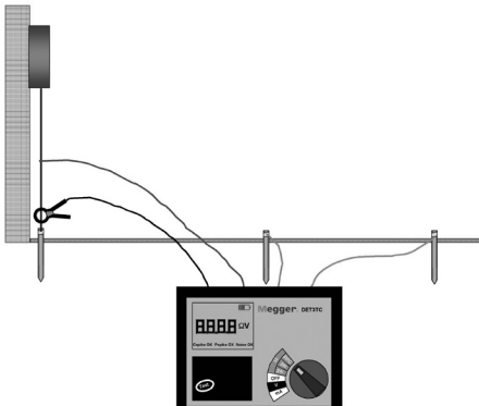
Abb. 27: Prüfen mit angeschlossener Elektrode (Attached Rod Technique, ART)
