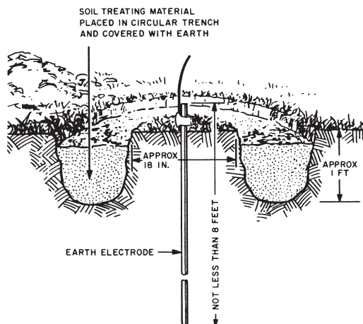
Abb. 19: Trench-Methode zur Bodenbehandlung 10
