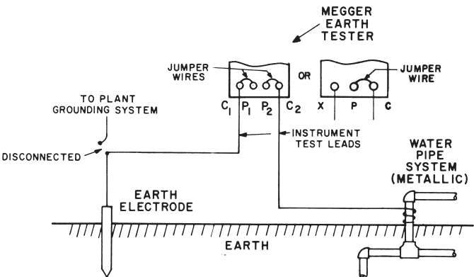
Abb. 12: „Dead Earth“-Methode oder Zweipunktprüfung des Erdungswiderstandes
