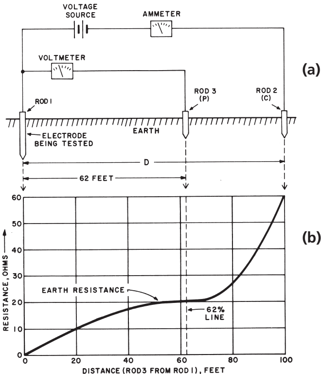
Abb. 10: Grundlagen zur Prüfung des Erdungswiderstandes
