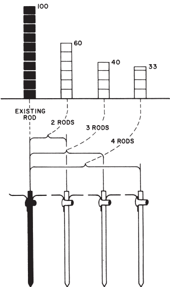
Abb. 17: Durchschnittliche Ergebnisse von Mehrstab-Erdungselektroden 8
