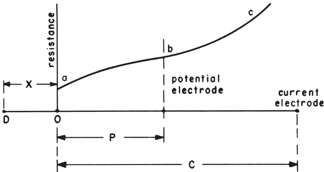
Abb. 28: Erdungswiderstandskurve für großflächige Systeme
