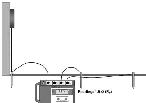
Abb. 25: Erdungswiderstandsmessungen
