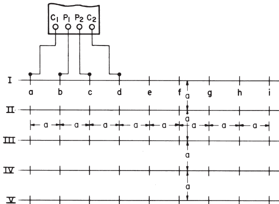
Abb. 5: Methode zur Erkundung der besten Erdungselektrodenposition bis zu einer Tiefe a . Die Position, die den niedrigsten Messwert auf dem Megger Erdungsprüfgerät liefert, ist am besten.
