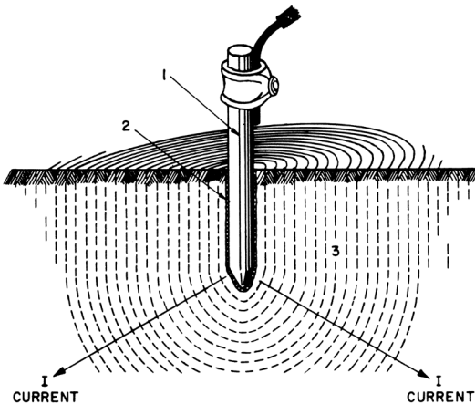
Abb. 9: Komponenten von Erdungswiderständen in einer Erdungselektrode
