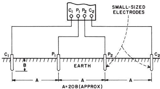
Abb. 1: Vierleitermessmethode zur Messung des Erdungswiderstandes
