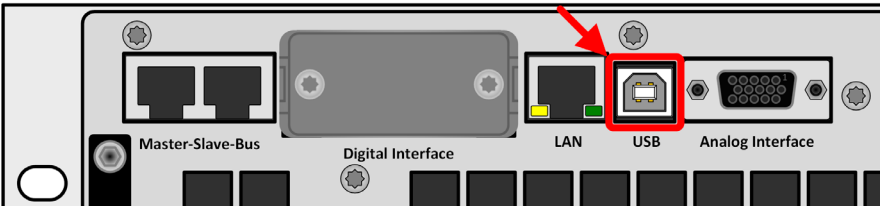
Bild 2 - USB-Port
