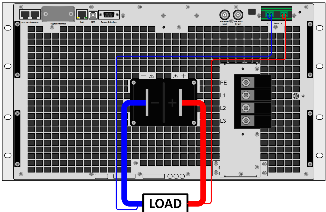
Bild 14 - Beispiel für eine Sense-Verdrahtung (DC- und Sense-Abdeckungen zu Zwecken der Veranschaulichung weggelassen)
