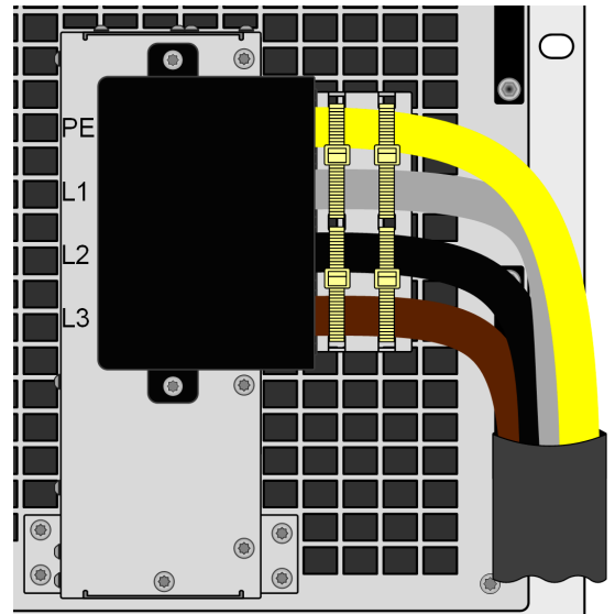
Bild 12 - Kompletter AC-Anschluß
