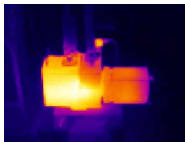
Vollständiges Wärmebild*
