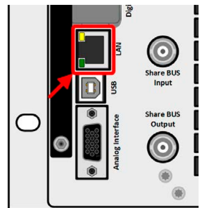
Bild 8 - LAN-Port
