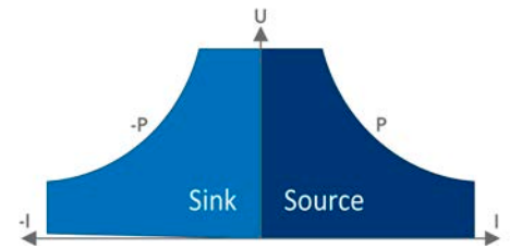
Bild 15 - Leistungsfläche 30 kW-Modelle
