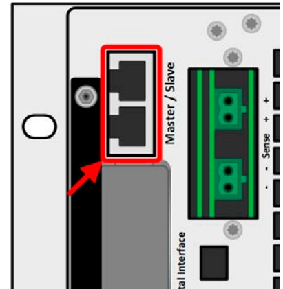
Bild 7 - Master-Slave-Busanschlüsse
