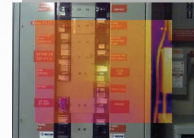
50 % Überblendung, Bild-in-Bild-Modus
