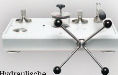
Hydraulische Vergleichstestpumpen P5514 und P5515 Siehe Seite 30
