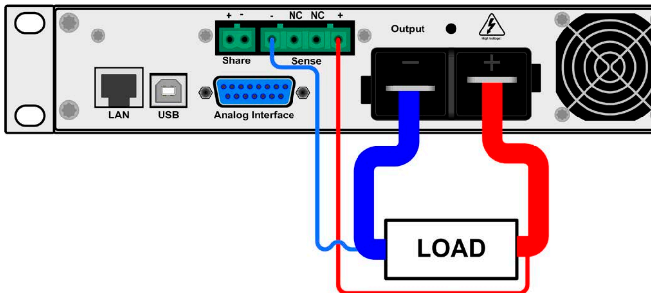
Bild 7 - Beispiel Fernfühlungsverdrahtung
