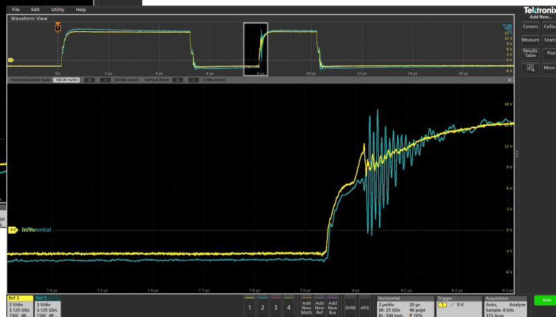
V_{GS} Turn-on
