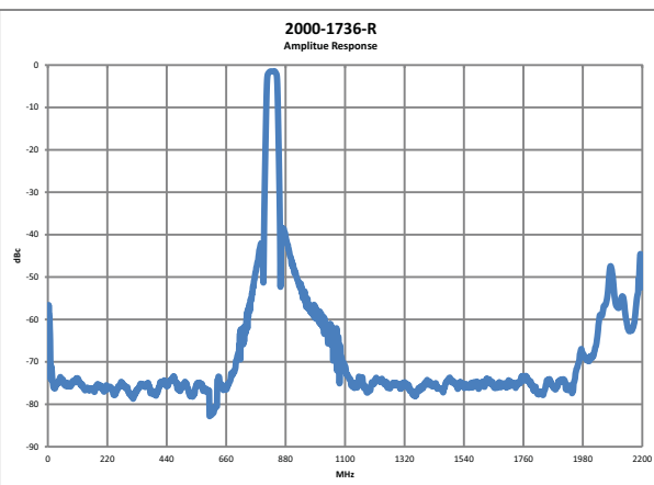
Stopband
