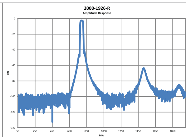
Stopband
