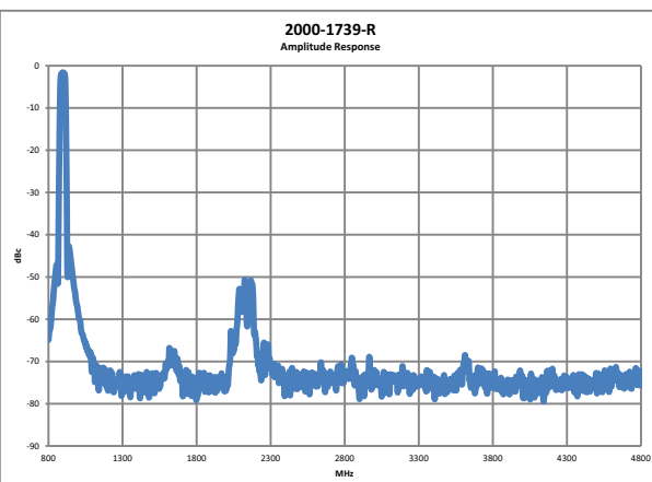
Stopband
