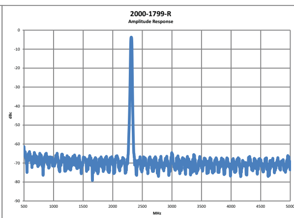
Stopband
