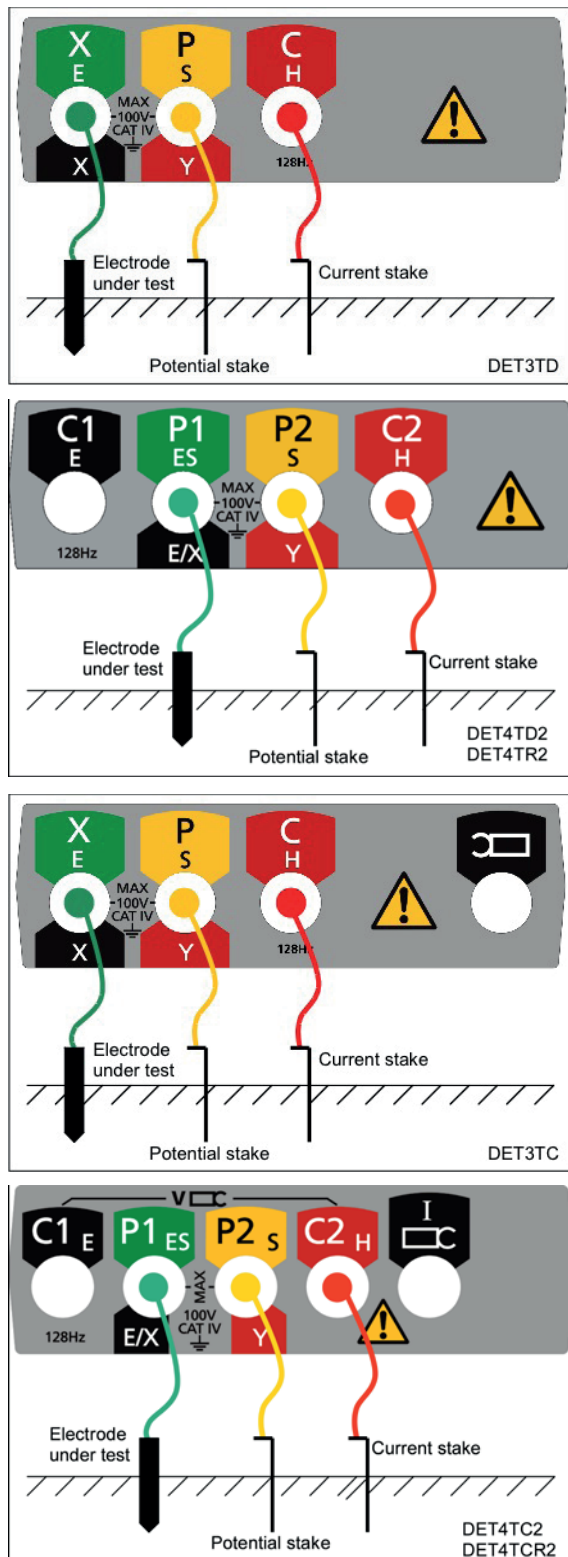
Abb. 18: Anschluss des Instruments zur 3-Klemmen-Widerstandsmessung
