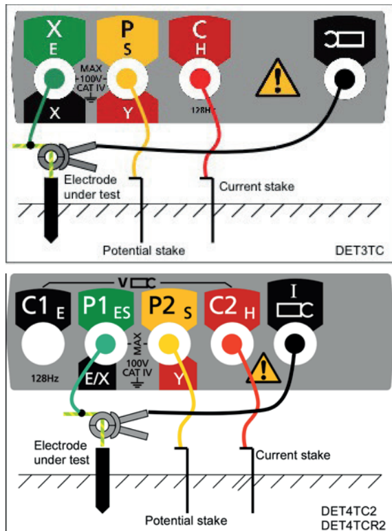
Abb. 31: Anschluss des Instruments zur 3-Klemmen-Widerstandsmessung mit ART
