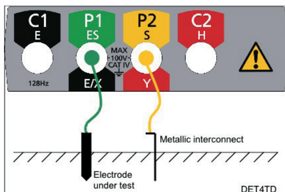
Abb. 13: Anschluss des Instruments zur 2-Klemmen-Widerstandsmessung
