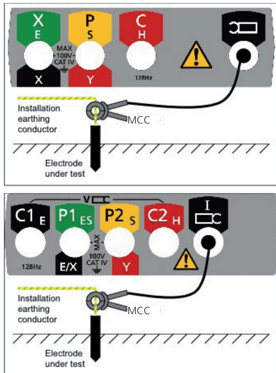
Abb. 29: Anschluss des Instruments zur Messung des Erdungsstroms
