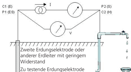
Abb. 3: Diagramm zur 2-Klemmen-Widerstandsmessung
