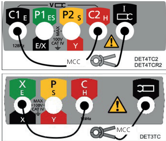
Abb. 37: MCC CLAMP-Nullkalibrierung
