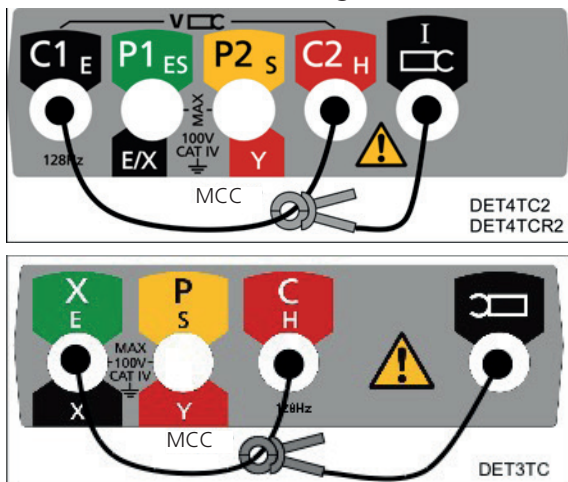
Abb. 38: 100%-Kalibrierung der MCC CLAMP
