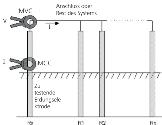
Abb. 7: Diagramm zur 2-Klemmen-Widerstandsmessung ohne Elektroden
