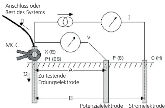
Abb. 6: Diagramm der 3-Klemmen-Widerstandsmessung mit ART ohne Nullabgleich
