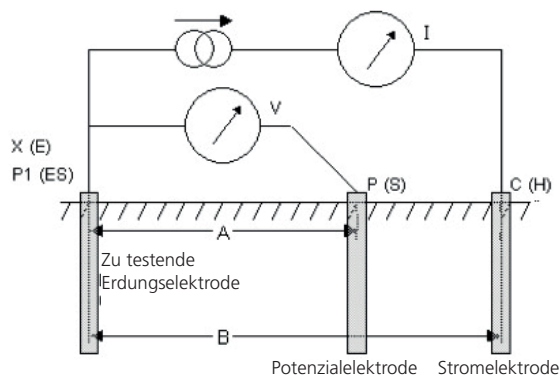
Abb. 5: Diagramm der 3-Klemmen-Widerstandsmessung ohne Nullabgleich
