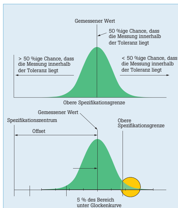
Abbildung 1. Der Offset der Glockenkurve für die Unsicherheit gibt an, wie Sie mit Schutzbereichen das für Kalibrierungen erforderliche Vertrauen erlangen.
