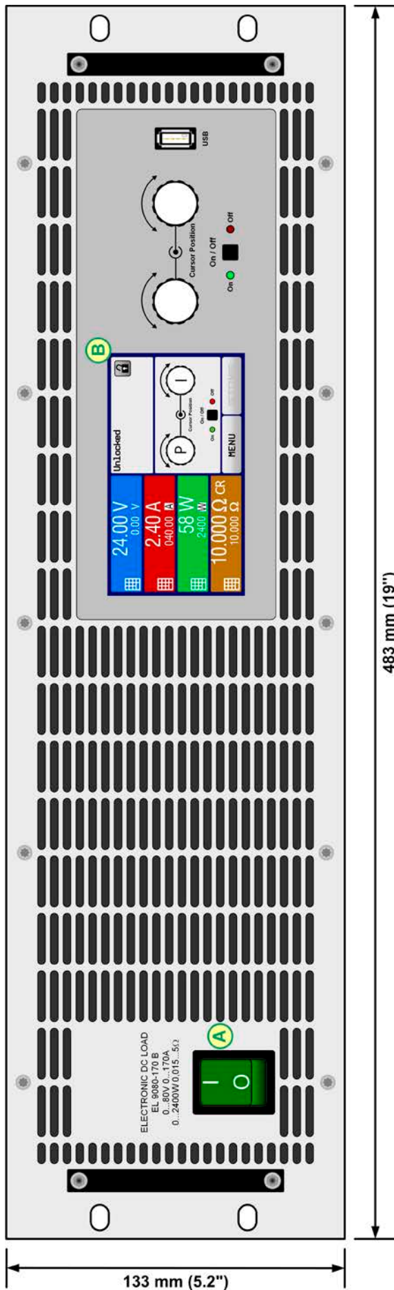
Bild 1 - Vorderansicht
