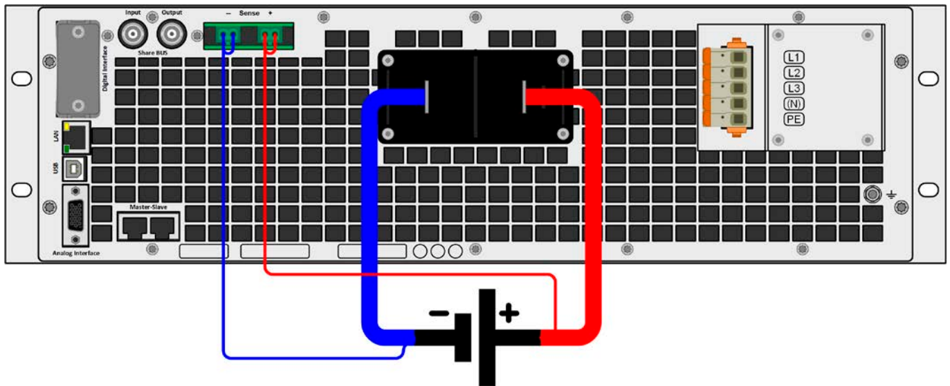
Bild 14 - Beispiel für eine Sense-Verdrahtung (DC- und Sense-Abdeckungen zu Zwecken der Veranschaulichung weggelassen)
