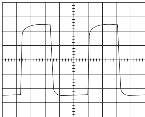
Unterkompensiert
