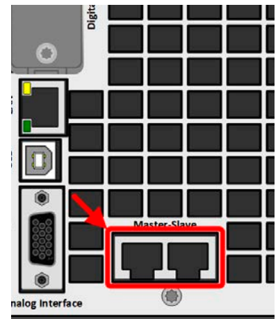
Bild 7 - Master-Slave-Busanschlüsse
