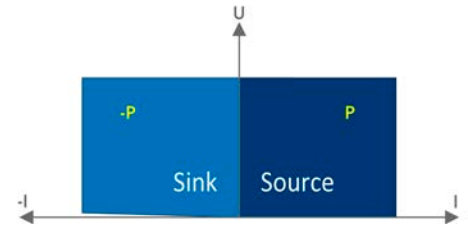
Bild 16 - Leistungsfläche 10 V-Modelle
