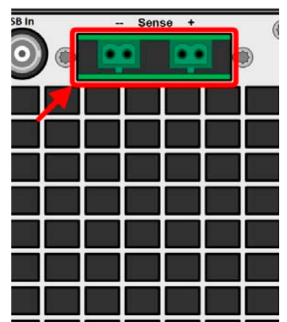
Bild 6 - Fernfühlungsanschlüsse
