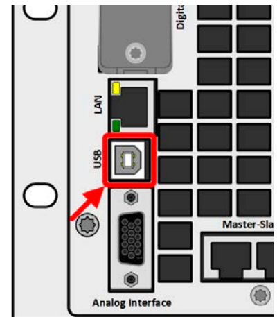
Bild 2 - USB-Anschluß
