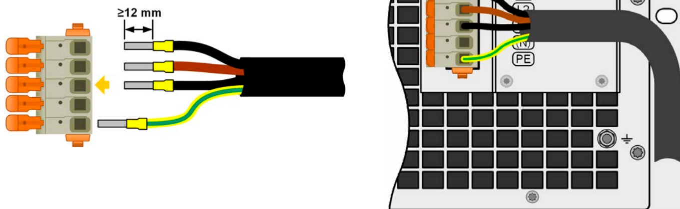
Bild 10 - Beispiel für ein Netzanschlußkabel mit 4 Adern für 10 kW und 15 kW (nicht im Lieferumfang enthalten)
