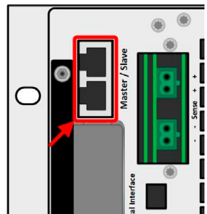
Bild 7 - Master-Slave-Busanschlüsse
