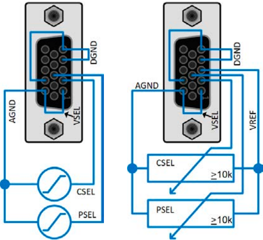
Beispiel mit ext. Spannungsquelle
