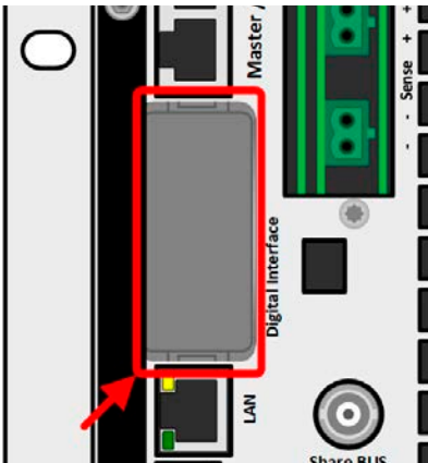
Bild 3 - Schnittstellenslot
