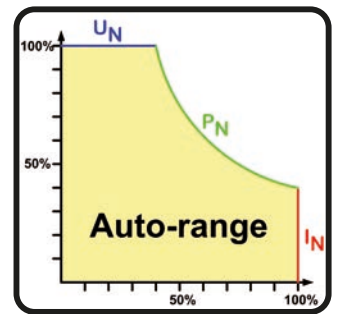
Bild 15 - Leistungsfläche
