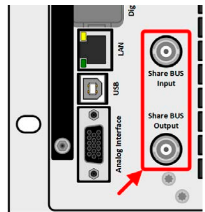
Bild 5 - Share-Bus
