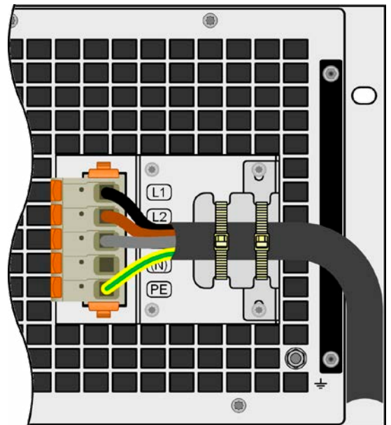
Bild 12 - Fertig montierte Zugentlastung
