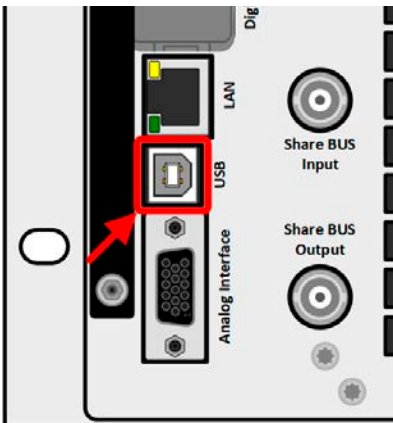
Bild 2 - USB-Anschluß
