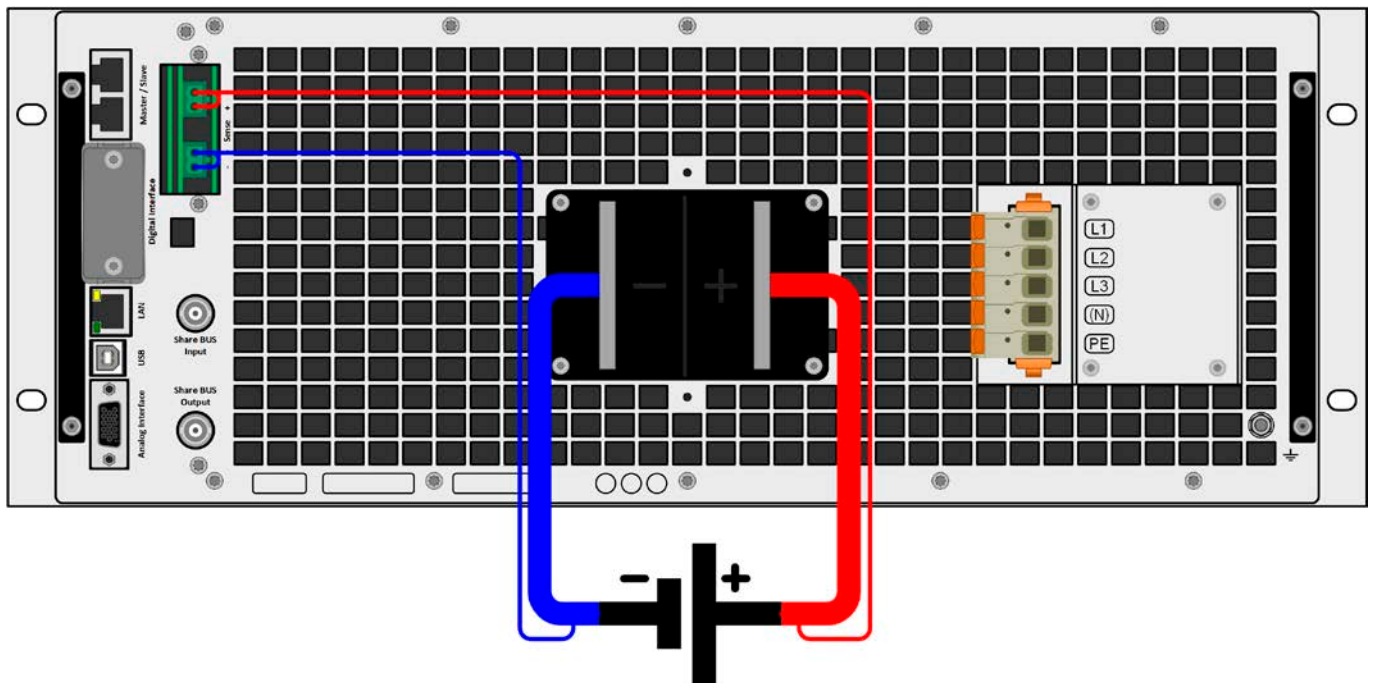
Bild 14 - Beispiel für eine Sense-Verdrahtung (DC- und Sense-Abdeckungen zu Zwecken der Veranschaulichung weggelassen)
