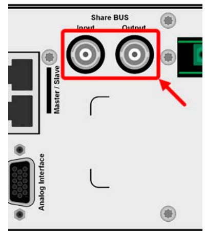
Bild 5 - Share-Bus
