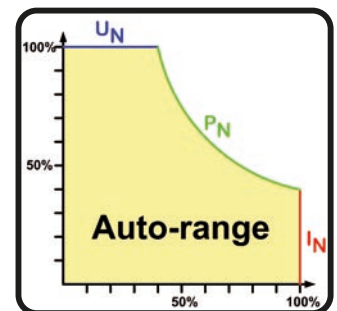
Bild 14 - Leistungsfläche
