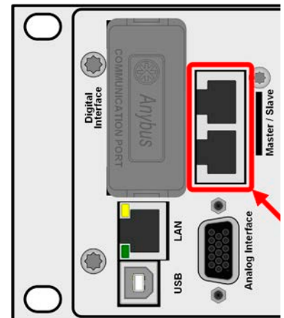
Bild 7 - Master-Slave-Busanschlüsse
