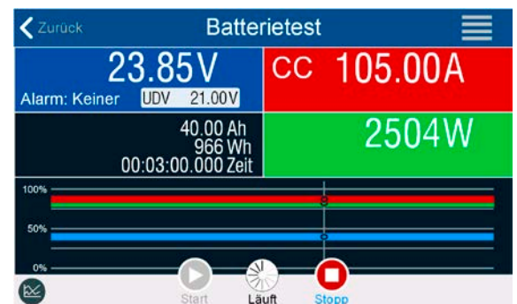
Bild 15 - Anzeigebeispiel vom statischen Entladen
