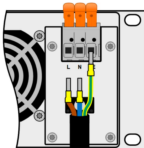
Bild 10 - Beispielkonfiguration eines AC-Kabels
