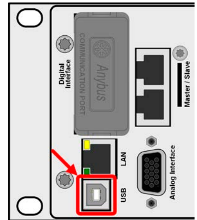
Bild 2 - USB-Anschluß
