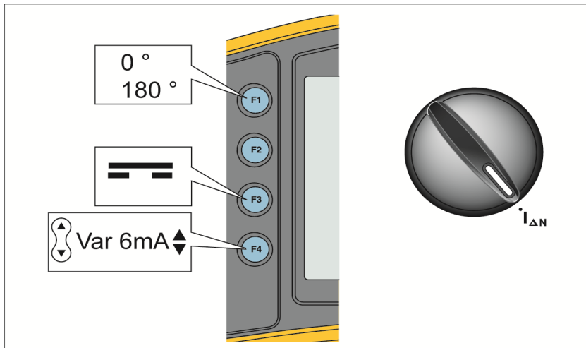
Abbildung 9. 6 mA RCD Typ A-EV or RDC-DD Auslösezeitmessung – VAR-Modus
