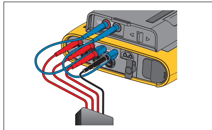
Abbildung 7. Messung mit Neutralleiterspannung und Gerätstromversorgung
