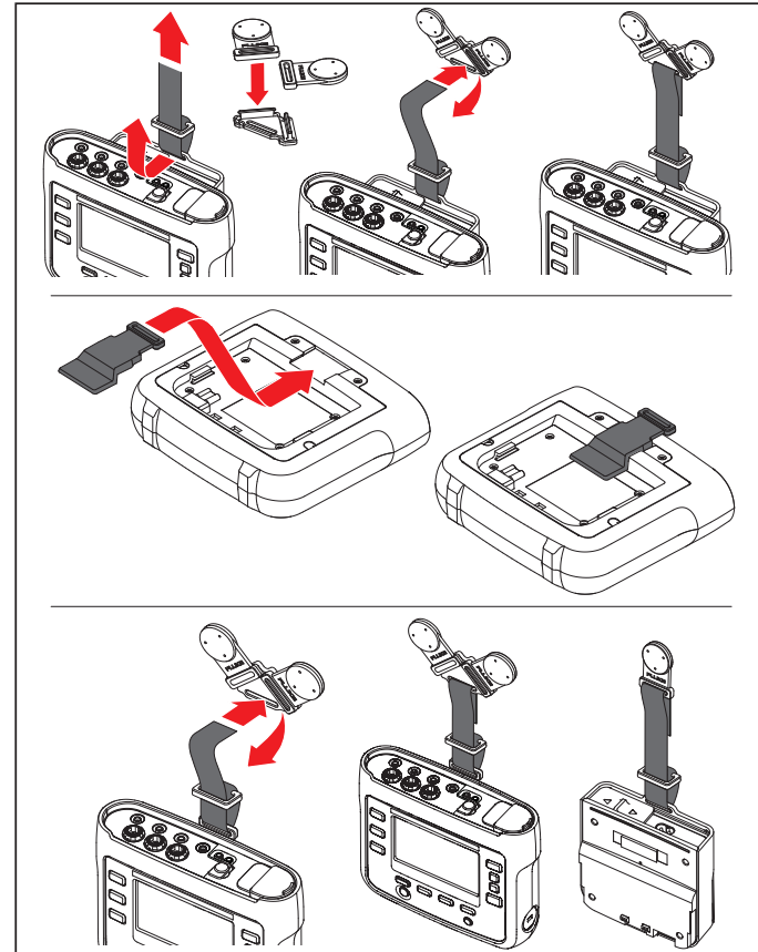
Abbildung 2. Magnethalterkit
