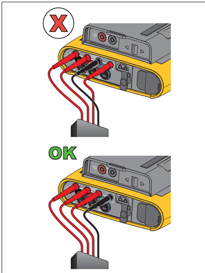
Abbildung 6. Messverbindung an Logger
