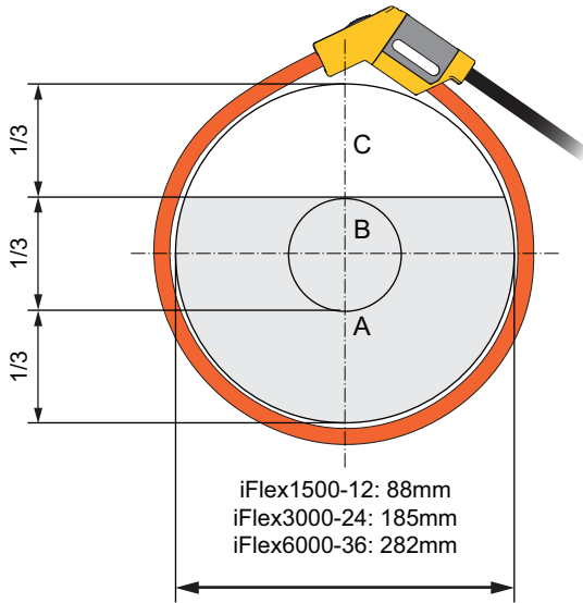
Abbildung 12. iFlex Messfühlerfenster
