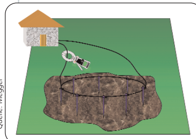
Bild 2: Erdung einer Schaltstation
