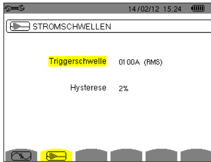
Abbildung 30: Bildschirm Anlaufstromgrenzwerte im Menü Anlaufstrommodus
