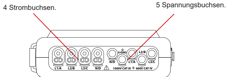
Abbildung 3: Anschlussbuchsen
