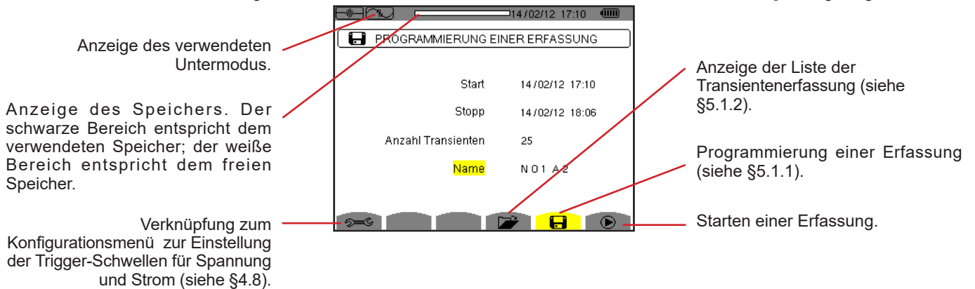
Abbildung 38: Bildschirm Programmierung einer Erfassung im Transienten-Modus
