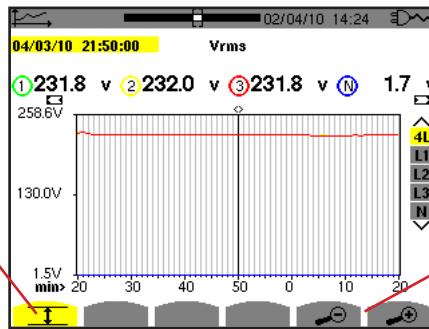
Abbildung 92: Vrms (4L) mit MIN-AVG-MAX
