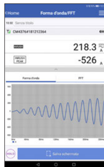
Forma d'onda/FFT
