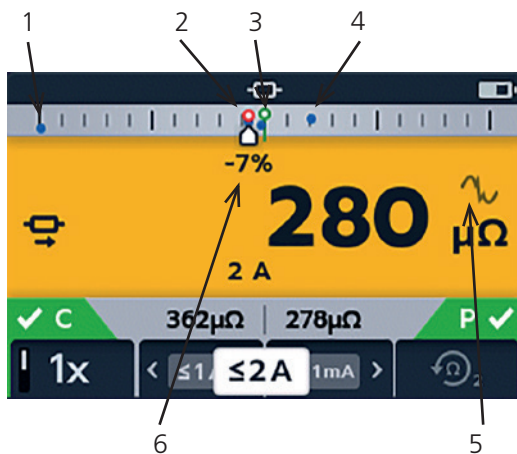
Farbanzeige des DLRO2 mit neuem Differenzmesser
