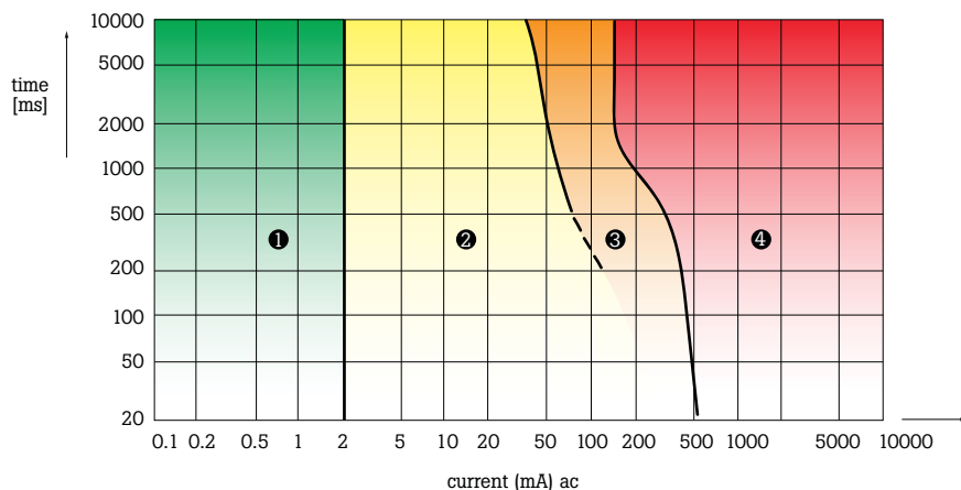
Abbildung 2: Auswirkung von Wechselstrom (bei Effektivwerten von 50 bis 60 Hz)
